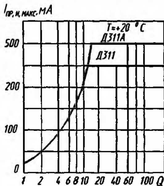
Зависимости максимального импульсного прямого тока от скважности
