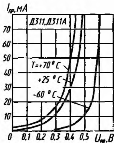
Зависимости прямого тока от прямого напряжения
