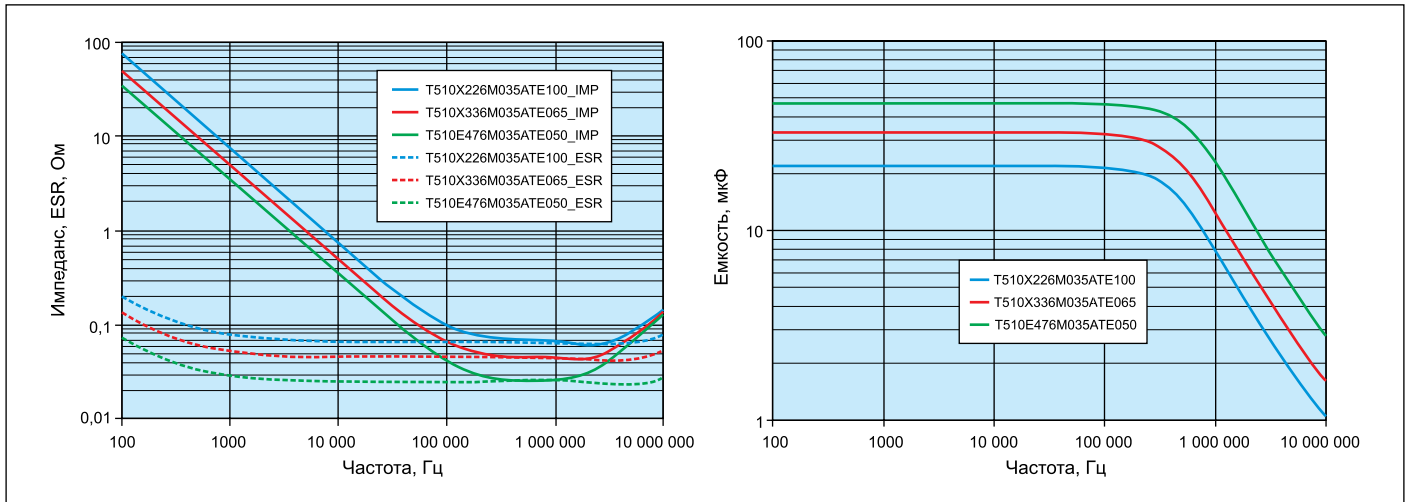
Рис. 6. Графики зависимости ESR и импеданса от частоты и емкости от частоты конденсаторов серии T510
