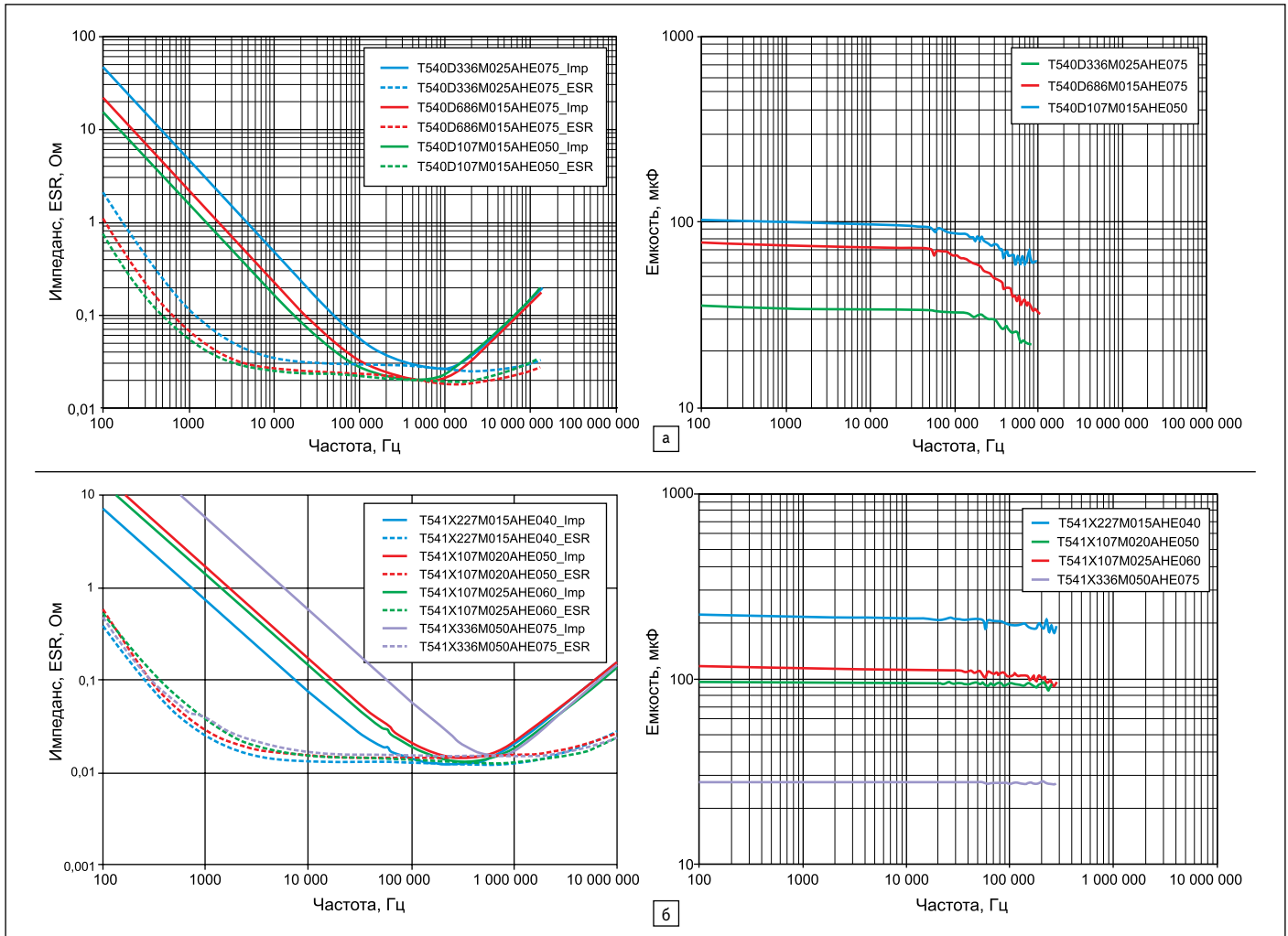
Рис. 8. Графики зависимости ESR и импеданса от частоты и емкости от частоты конденсаторов серий: а) T540; б) T541
