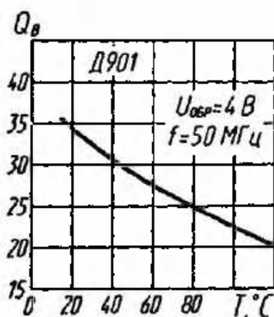
Зависимость добротности от температуры
