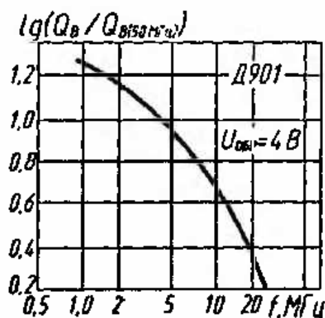
Зависимость относительной добротности от частоты
