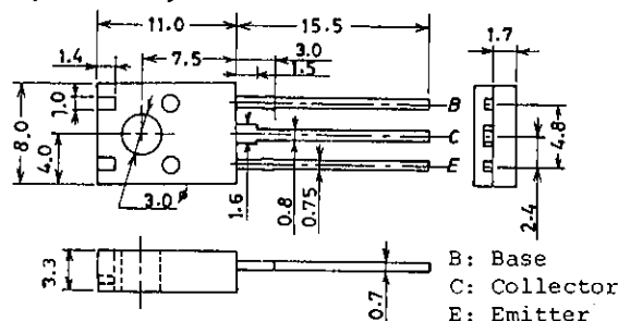
Package Dimensions 2042A (unit:mm)
