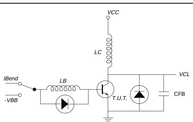
Fig.15. Test Circuit RBSOA.
