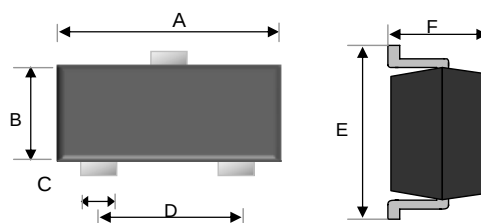
SOT-323
