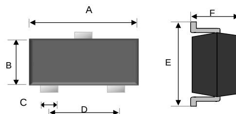
SOT-723
