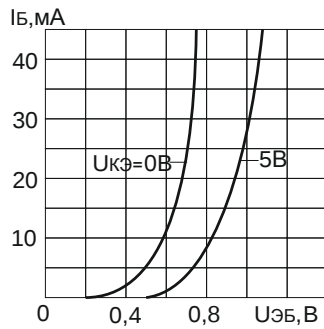
Входные характеристики
