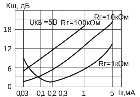
Зависимость коэффициента шума от тока коллектора КТ3107 А-Д,И,К
