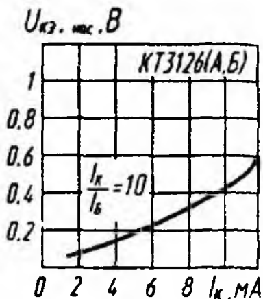
Зависимость напряжения насыщения коллектор—эмиттер от тока коллектора
