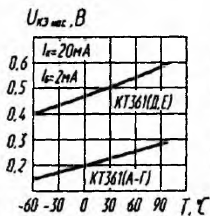
Зависимости напряжения насыщения коллектор—эмиттер от температуры
