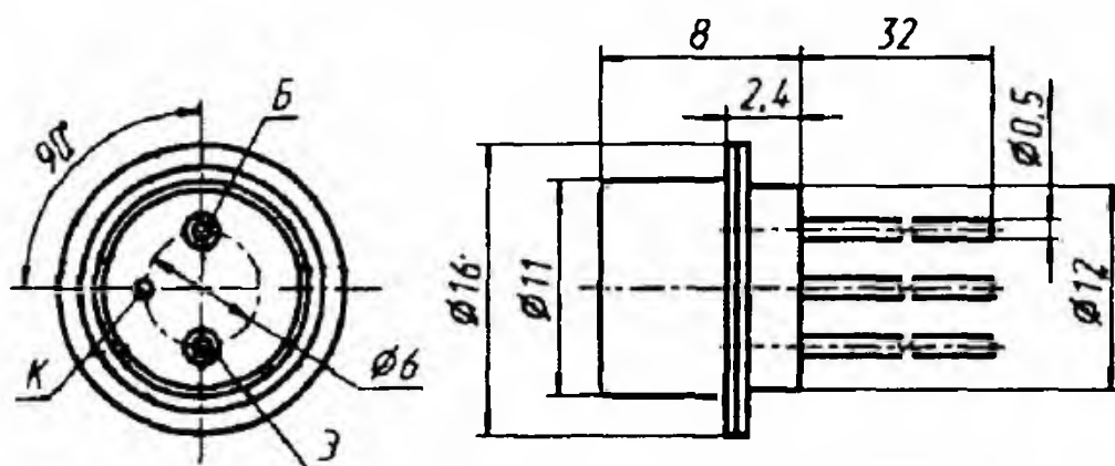
КТ604(А,Б)
