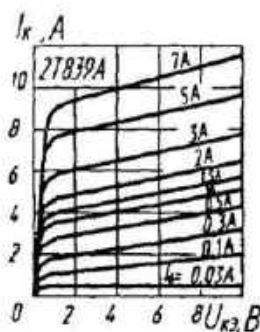
Выходные характеристики
