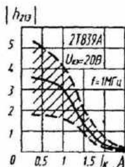
Зона возможных положений зависимости модуля коэффициента передачи тока от тока коллектора
