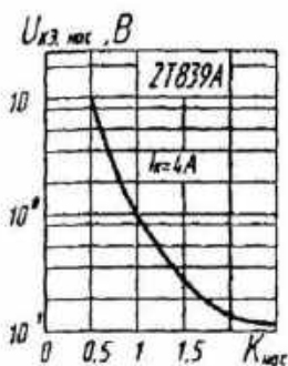
Зависимость напряжения насыщения коллектор—эмиттер от коэффициента насыщения
