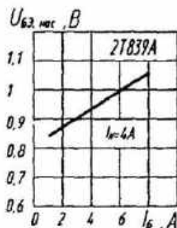
Зависимость напряжения насыщения база—эмиттер от тока базы
