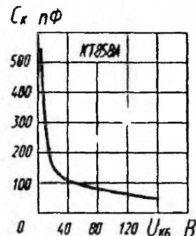
Зависимость емкости коллекторного перехода от напряжения коллектор—база
