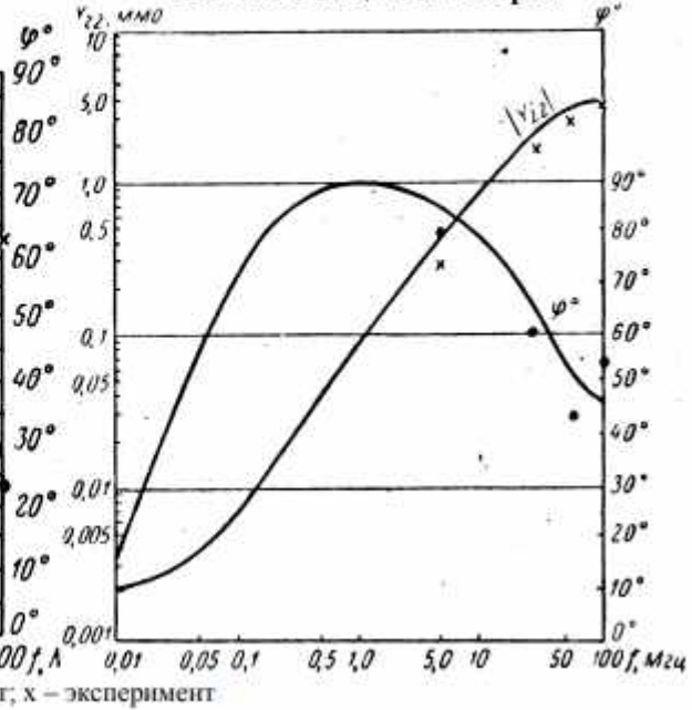
Частотная зависимость Y_{22} (П403) в схеме с общим эмиттером
