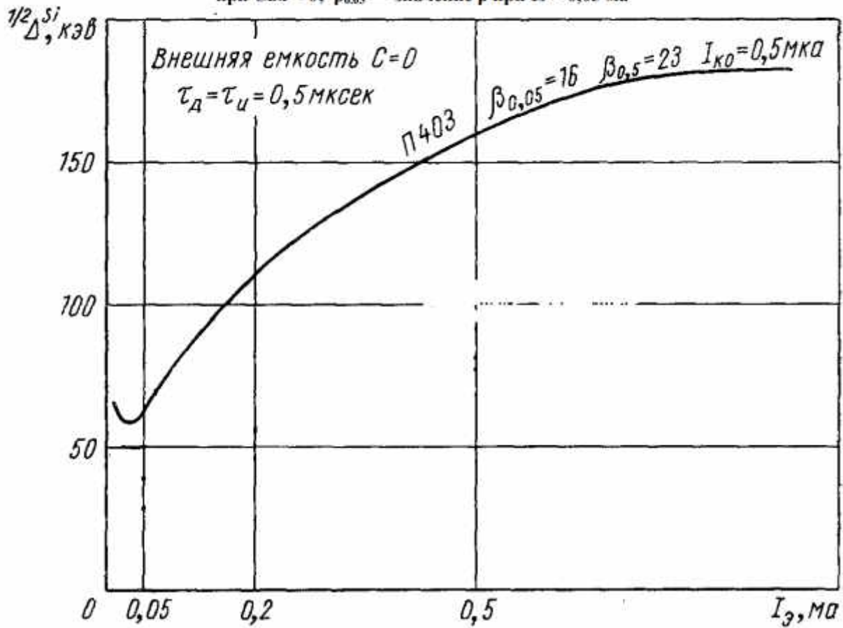
Экспериментальные шумовые характеристики транзисторов при S_{вх} = 0 ; \beta_{0,05} — значение \beta при I_3 = 0,05 ма
