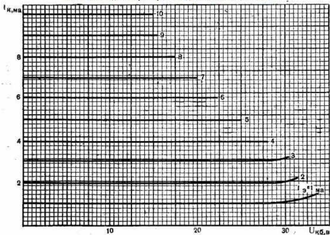
типовые выходные характеристики для схемы с общей базой
