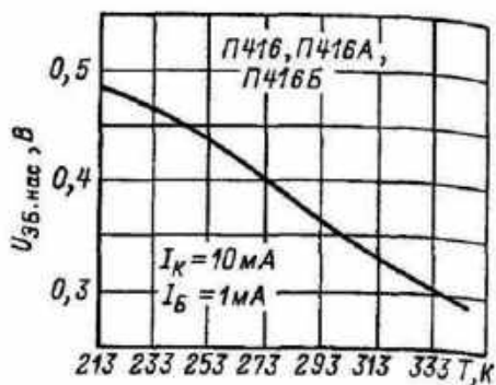
Зависимость напряжения насыщения эмиттер-база от температуры.
