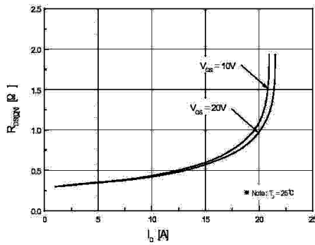
R_{DS(ON)} - I_D
