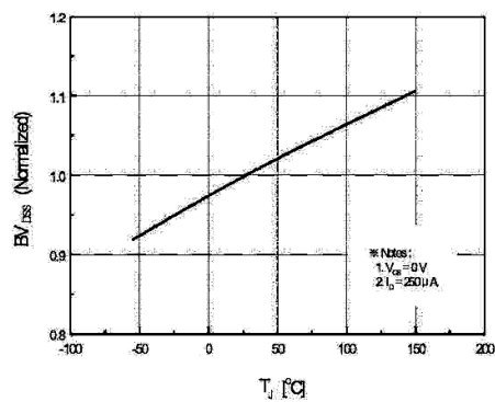
BV_{DSS} - T_J
