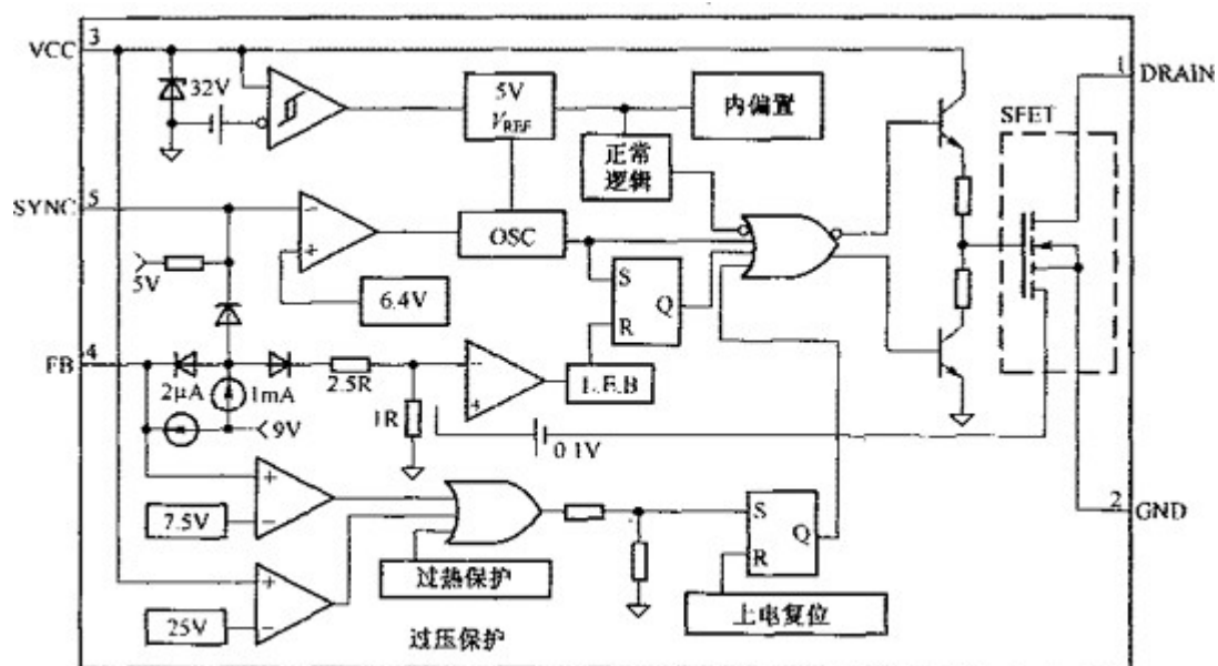
图 4-4 DP104C 内部电路框图
